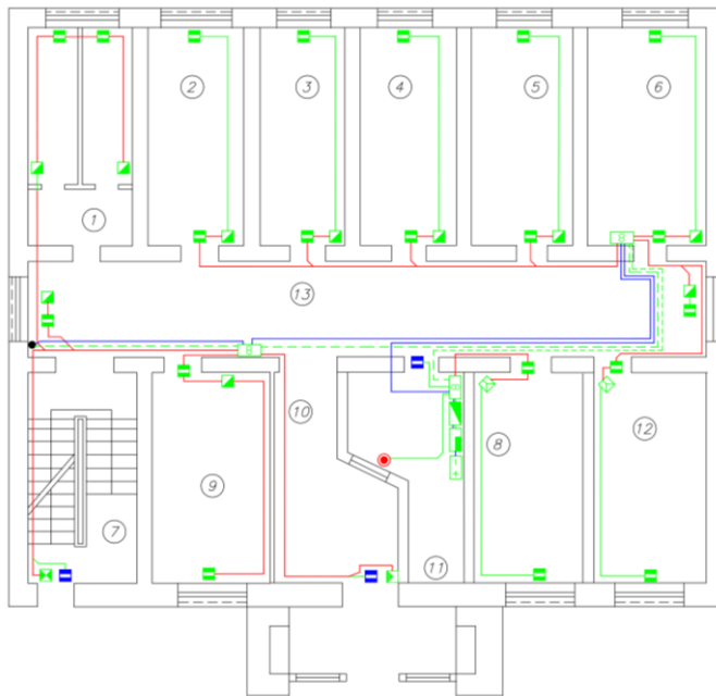
Экспликация помещений
